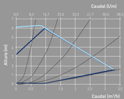
Curva del circulador incluido en el Kit para 2º circuito.
