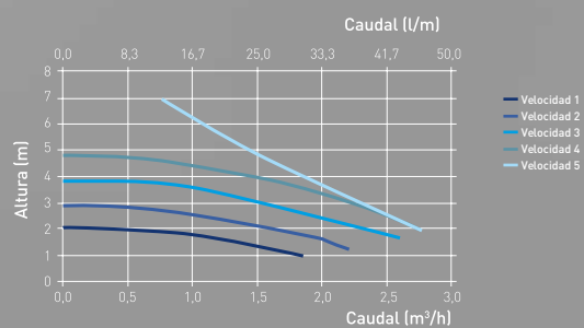
Curva del circulador incluido en el Kit para 2º circuito.
