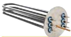
RESISTENCIA "RB": Resistencia bridada para modelos GEISER INOX de "SIMPLE PARED", ACUMULACIÓN y SERPENTÍN
